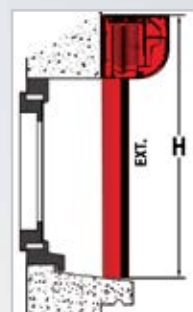
Pose en façade ou en applique
