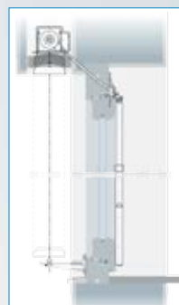
POSE : en niche, lames ourlées 80, treuil GUIDAGE : câbles
